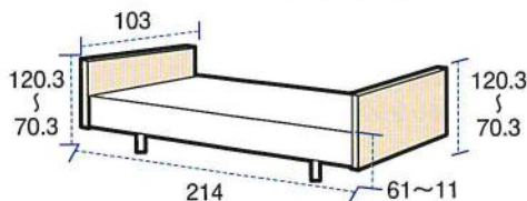
ベッド寸法図 (cm)
