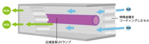
● NCCセルの構造
